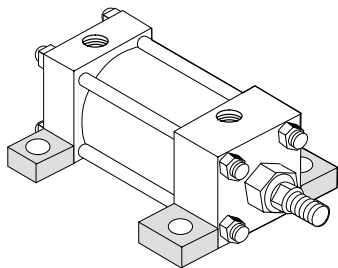
Code 01 (MS2) Side Lug
